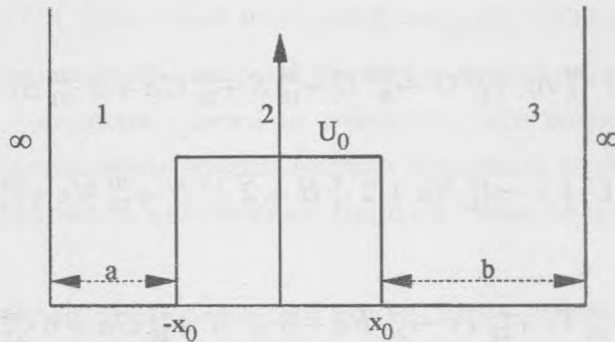
Рис. 1. Потенциальная яма.
