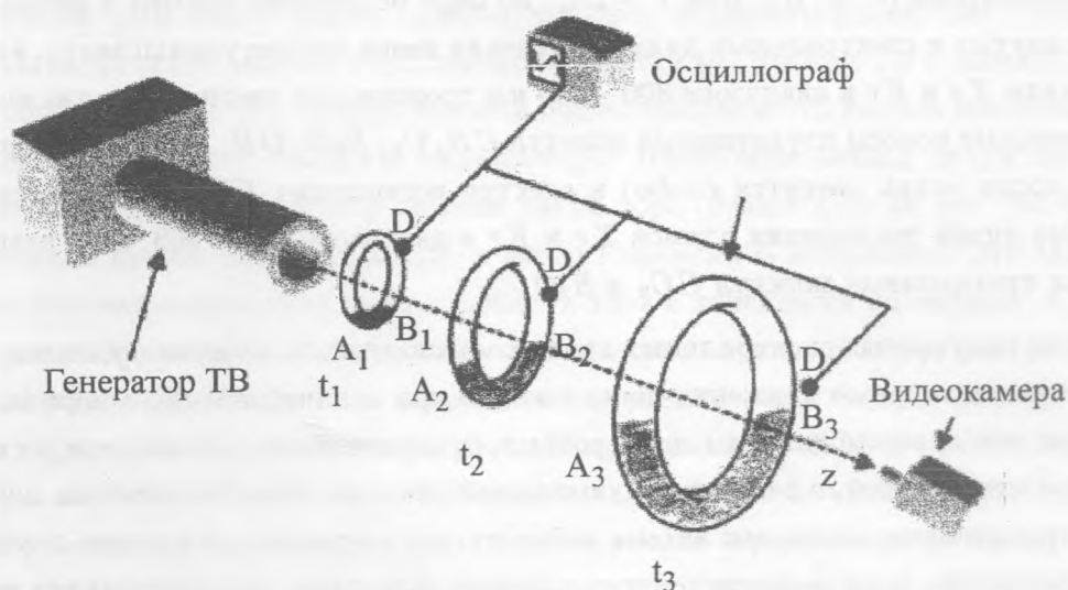
Рис. 1. Взаимное расположение элементов экспериментальной установки и вихря в различные моменты времени. D – акустические датчики.
