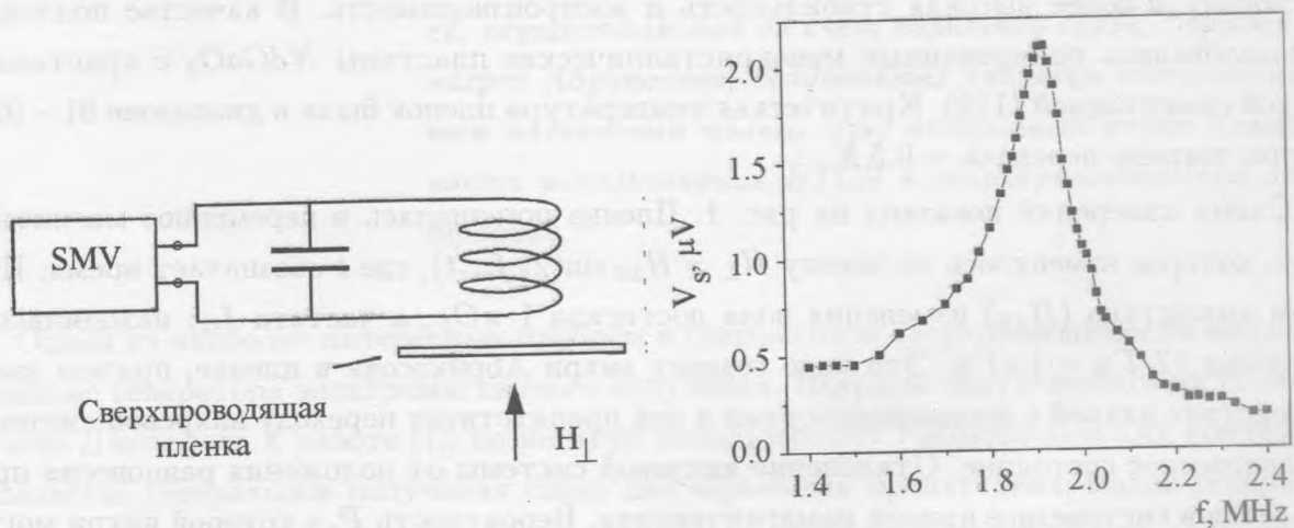
Рис. 1. Схема измерений, SMV – селективный микровольтметр.
