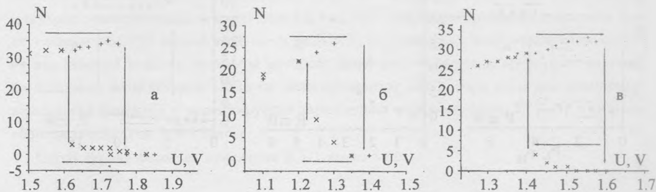
Рис. 2. Экспериментальные (+, x) зависимости числа абберационных колец самофокусировки в световом пучке, прошедшем планарный НЖК (ЖКМ-1282 + 0.025% КД-1, толщина L = 100 мкм, \lambda = 532 нм, угол падения \alpha = 52^\circ ), от приложенного низкочастотного (3 кГц) напряжения U при различных значениях смещения НЖК из фокальной плоскости \Delta и мощности светового пучка: (а) \Delta = 0 , P = 8 мВт; (б) \Delta = 16 см, P = 4 мВт; (в) \Delta = 16 см, P = 8 мВт.
