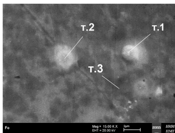
Рис. 4: Фотография поверхности медной пленки на Fe, полученная с помощью сканирующего электронного микроскопа. В точках “T.1”, “T.2” и “T.3” снимались рентгеновские спектры.
